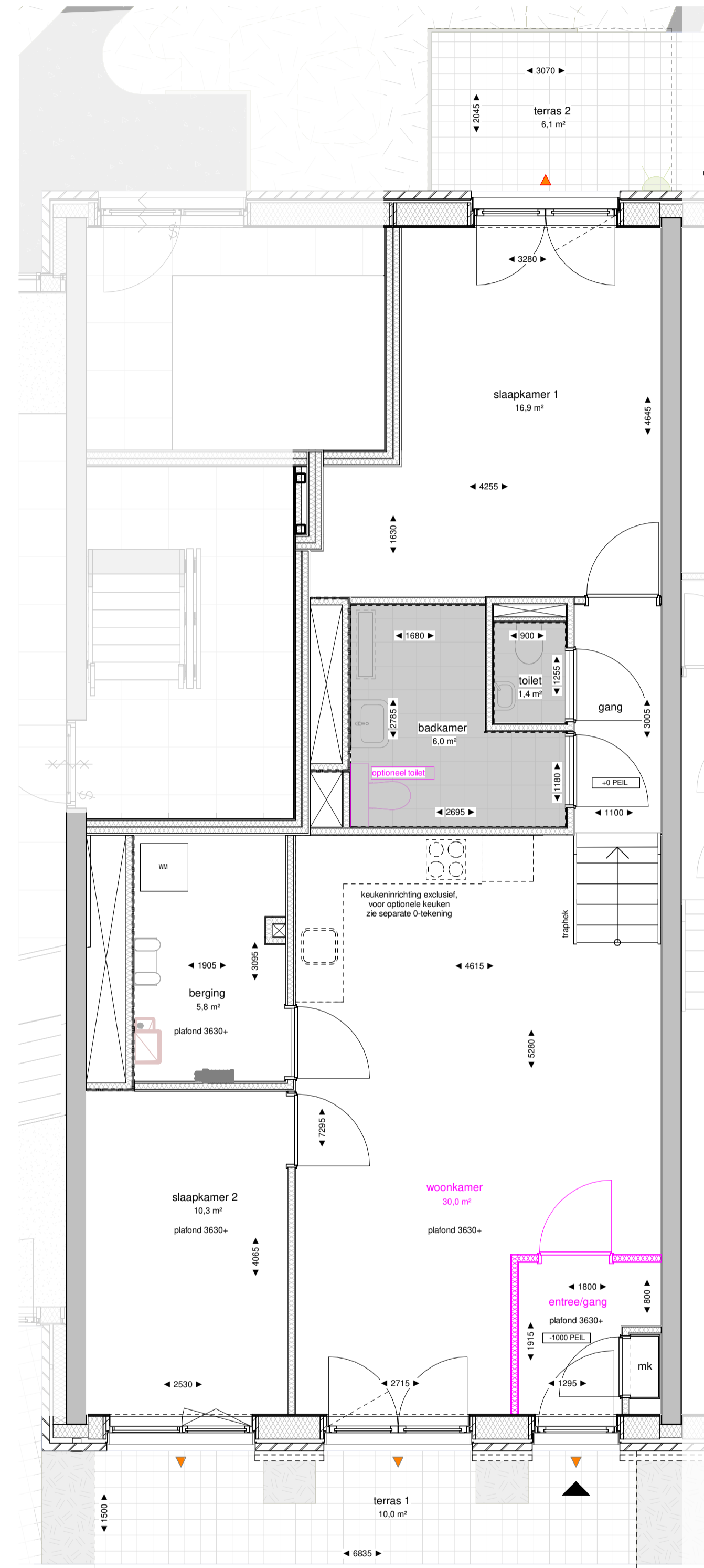
J.00.05 begane grond optie schaal 1 : 50
