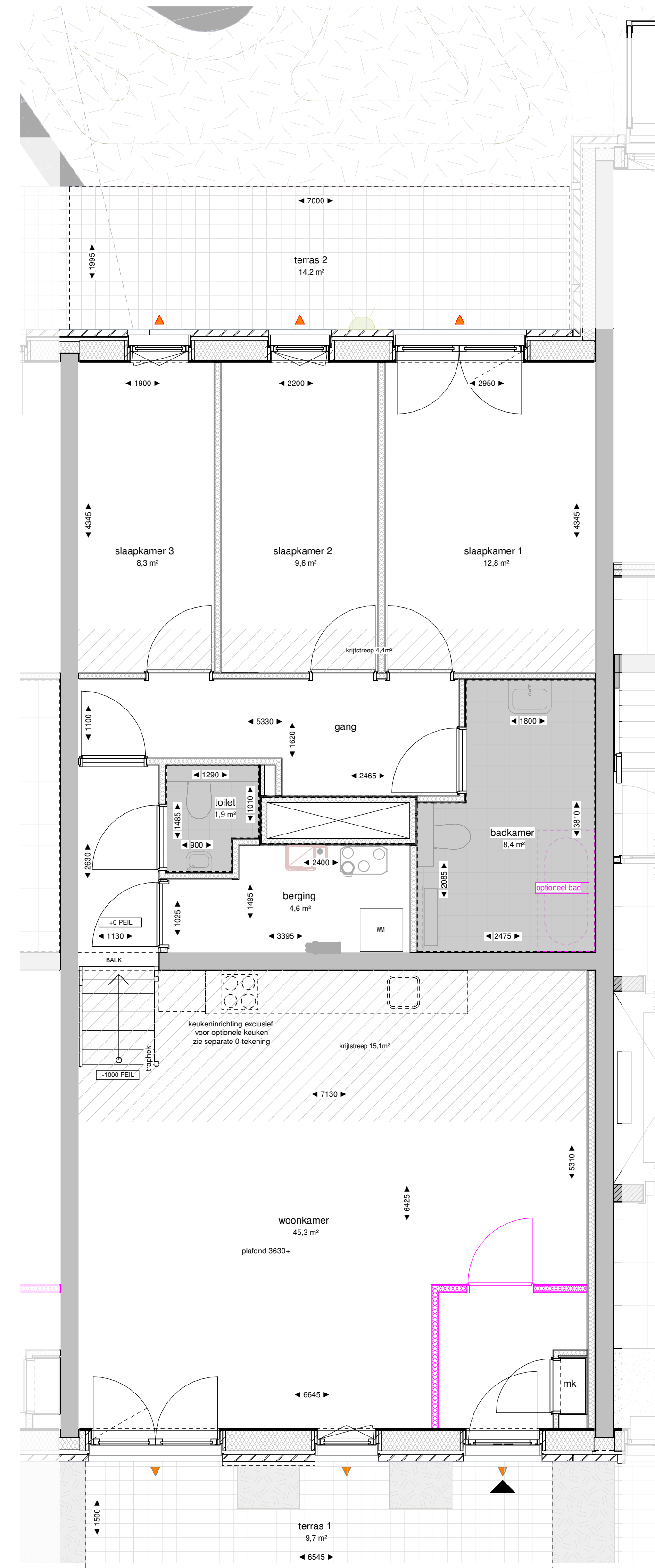
I.00.01 begane grond optie schaal 1 : 50
