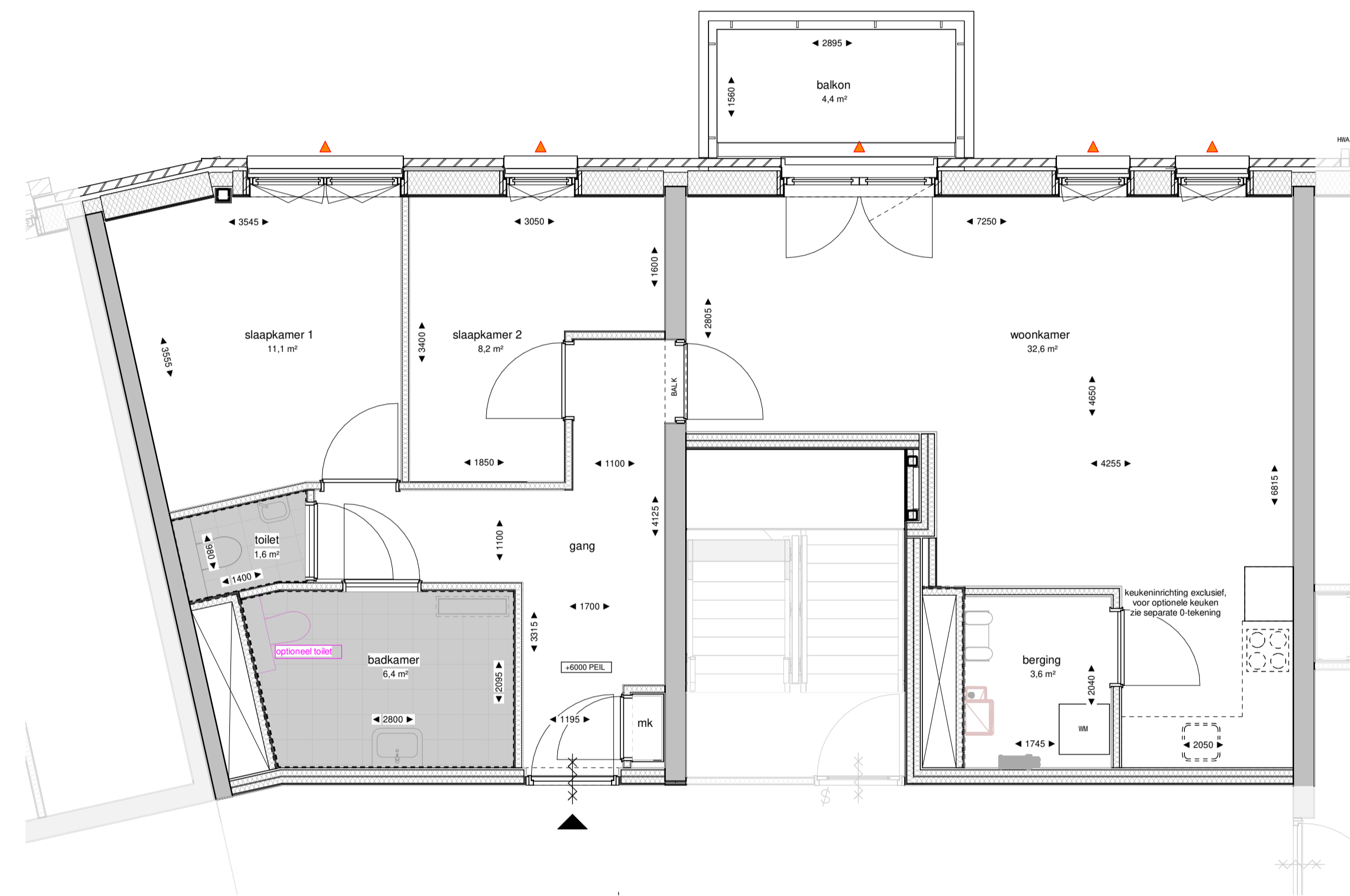
J.02.06 tweede verdieping optie schaal 1 : 50
