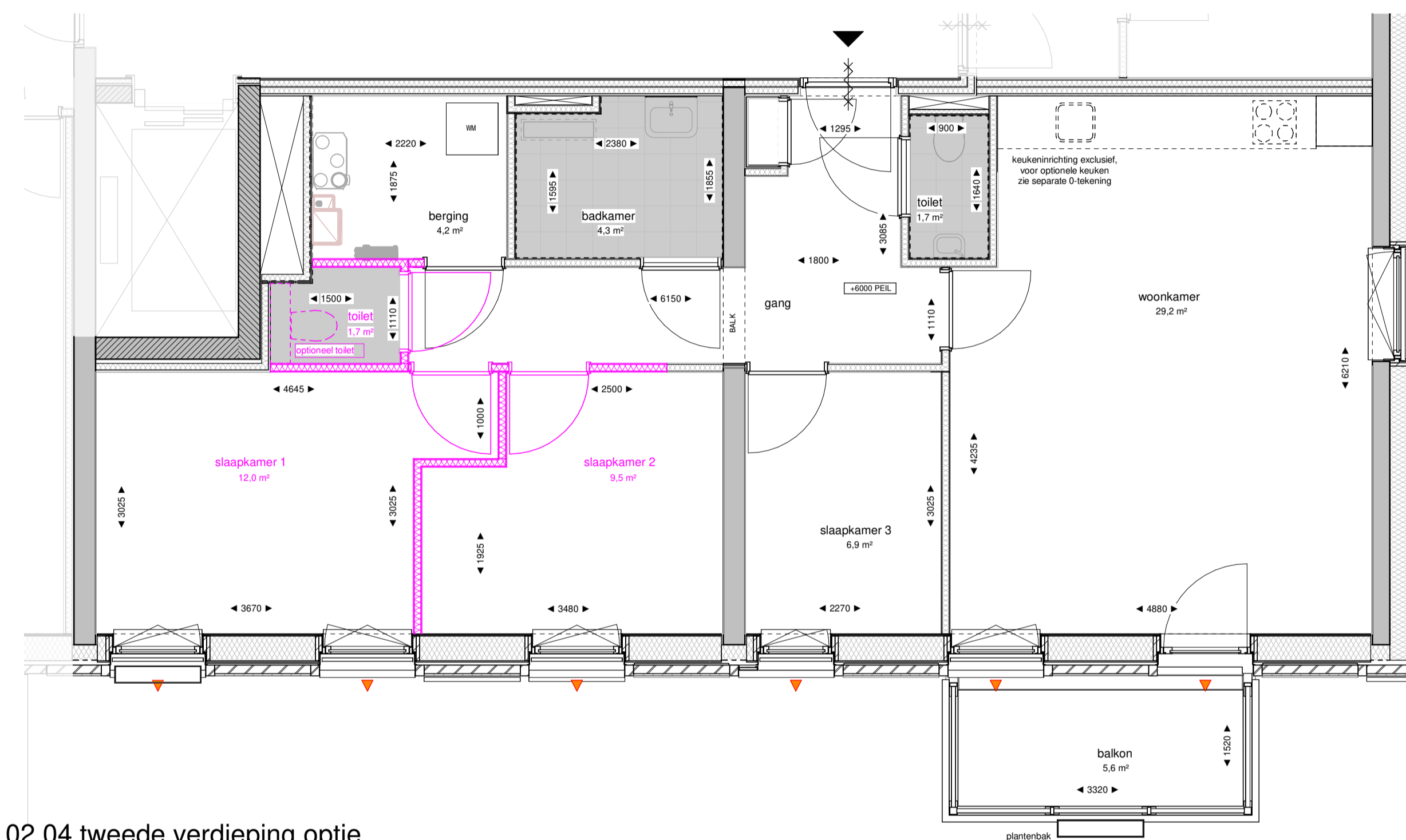
I.02.04 tweede verdieping optie schaal 1 : 50
